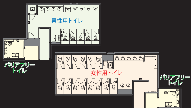
6F 大ホールトイレ平面図
