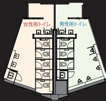
平面図
