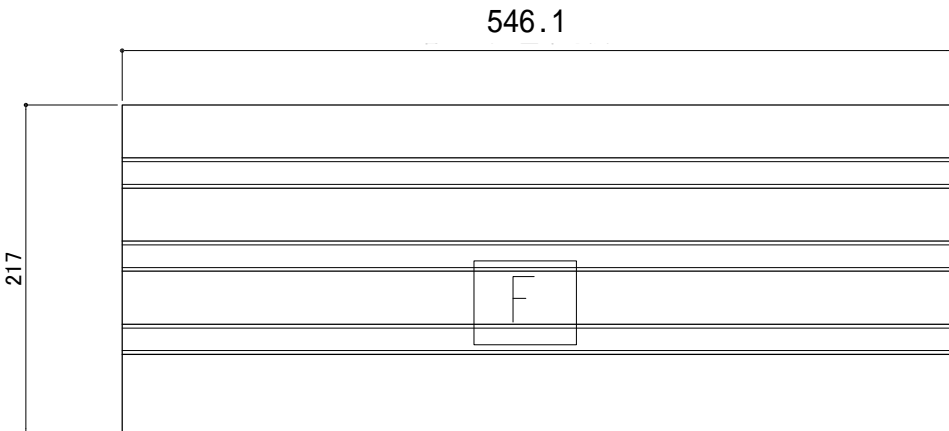
PC打込柱型テラコッタタイル形状図
