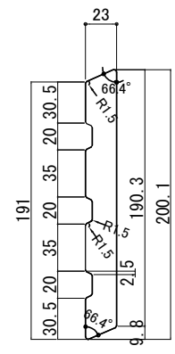
PC打込梁型テラコッタタイル形状図
