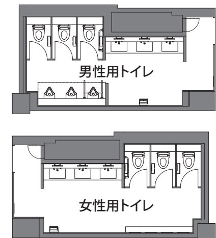
改修後 平面図
