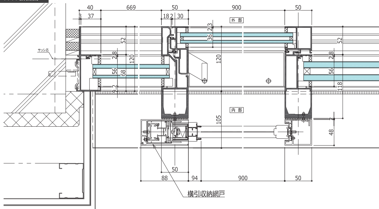
A-A 断面図
