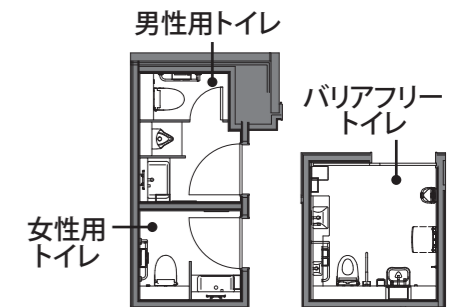
1Fトイレ 平面図
