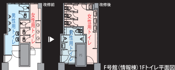
F号館(情報棟)1Fトイレ平面図
