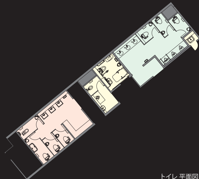
トイレ 平面図
