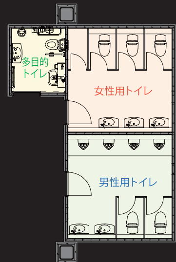
トイレ 平面図
