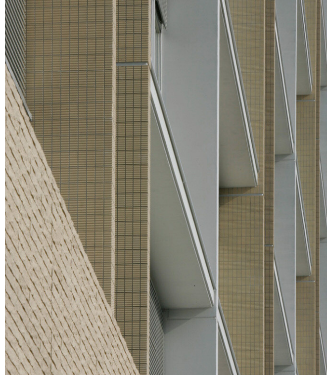
南西側タイルディテール
