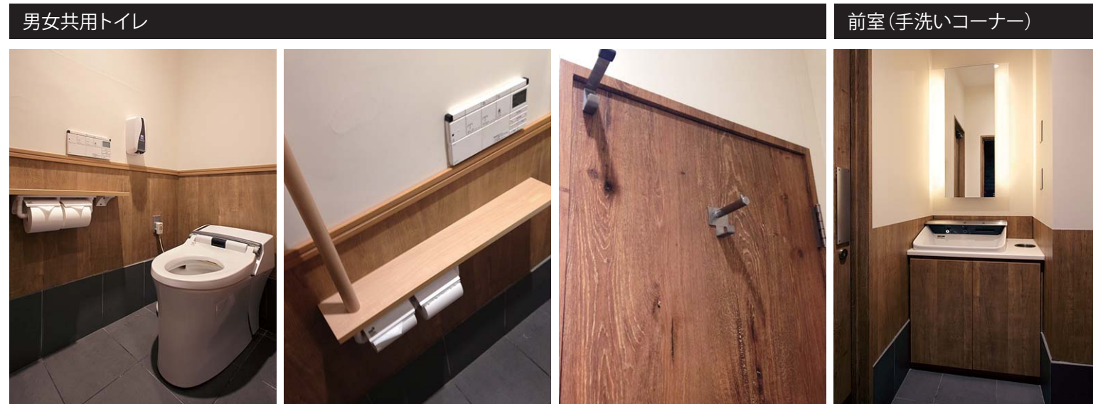
タンクレストイレを採用し、コンパクトでも動作空間を確保。室内は小物を置ける棚と手すりが一体となった「棚手すり」の設置でスッキリとした空間となっている。ドアには戸当たりとは別にダブルフックを設置、手荷物にも配慮。食事前後の手洗いが快適に行えるよう、個室の外に多機能洗面器を設置。
