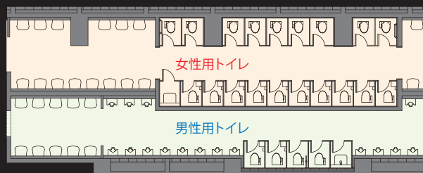
1F大ホールトイレ 平面図
