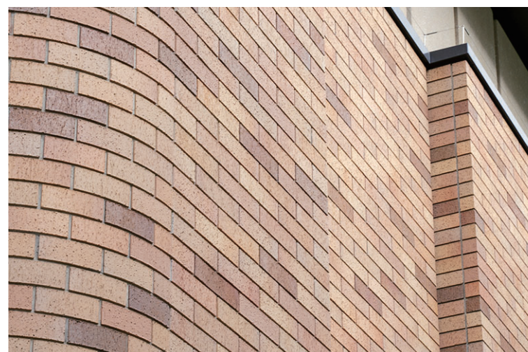
外装壁面タイルディテール(コーナー部)
