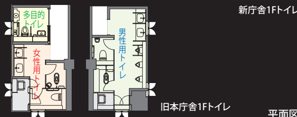
平面図
