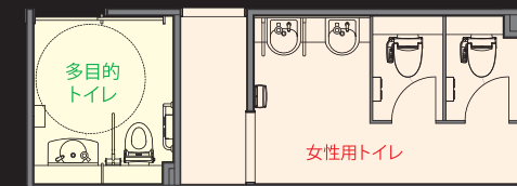
トイレ 平面図
