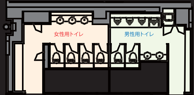
児童用男女トイレ平面図
