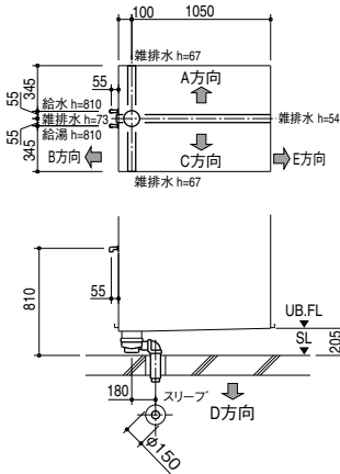
※シャワーユニットの給排水位置
